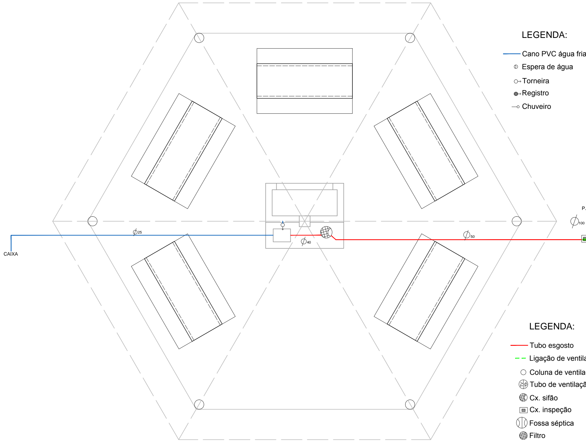
Projeto Hidrossanitário
