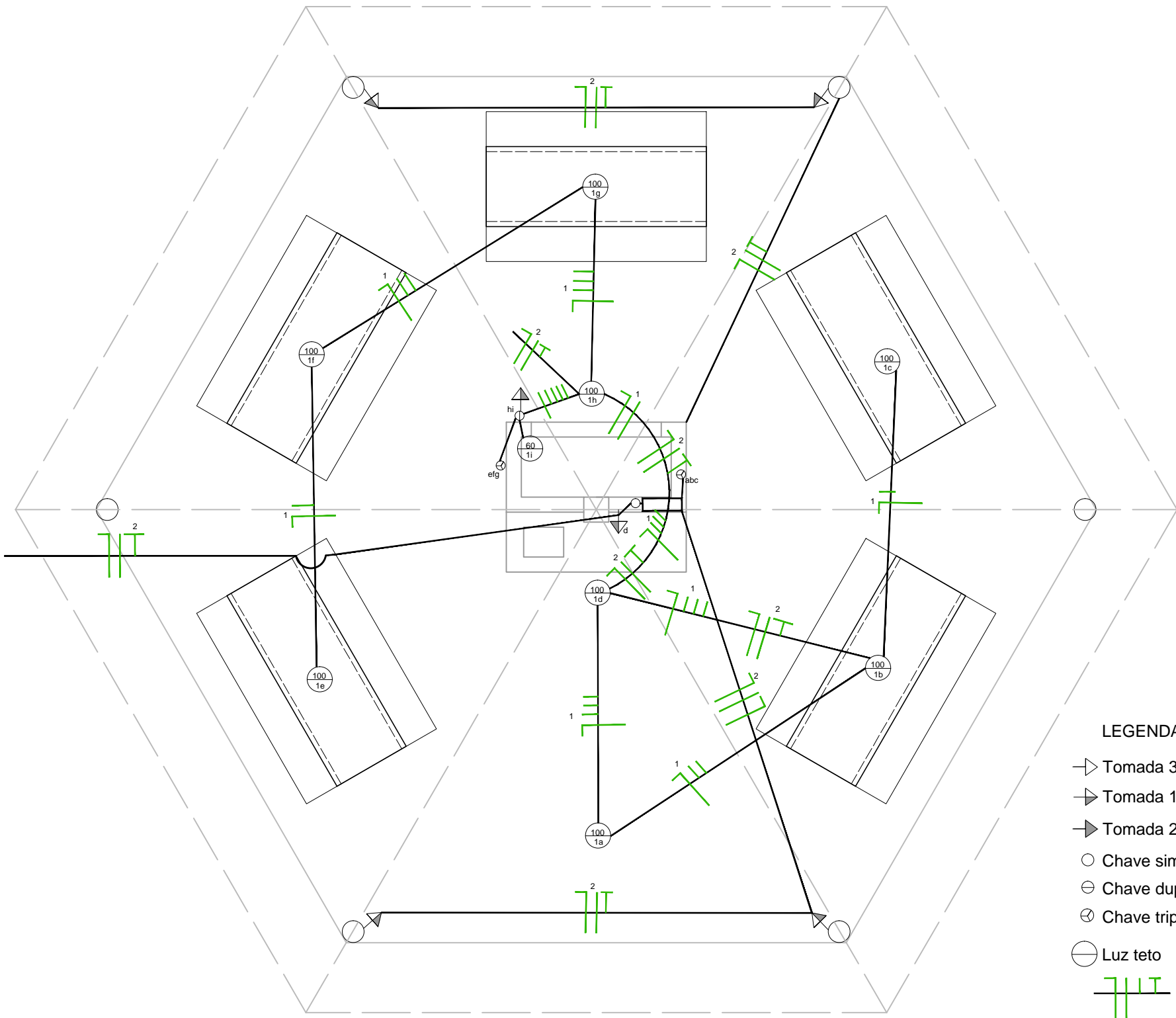
Projeto Elétrico
