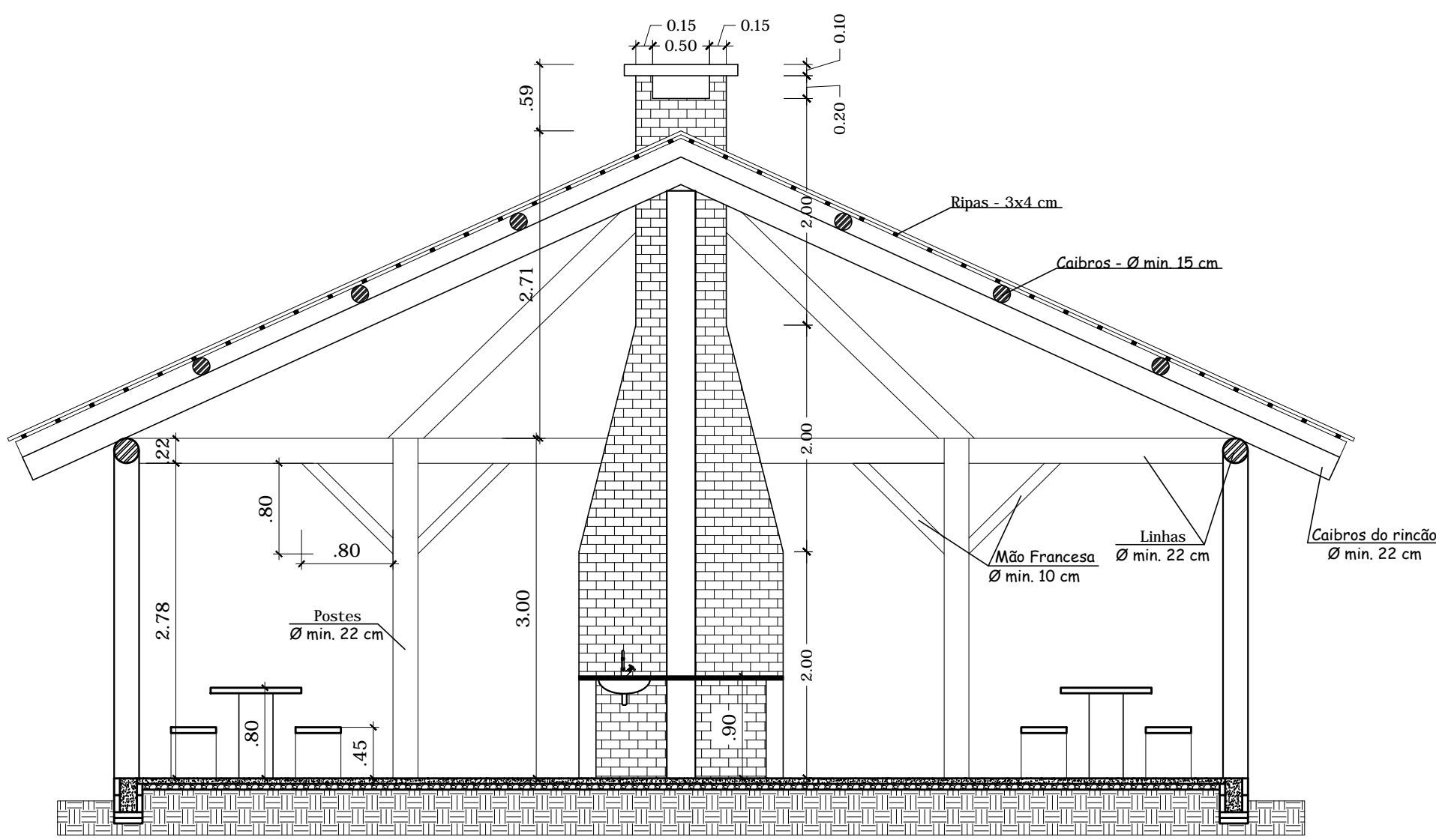
Corte A-A
